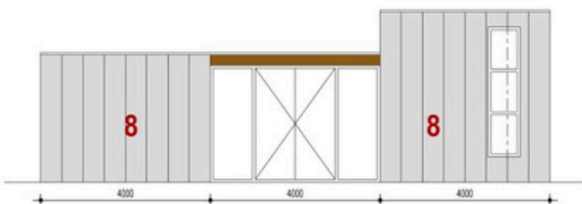
Zuidgevel
