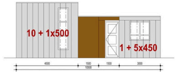
Oostgevel
